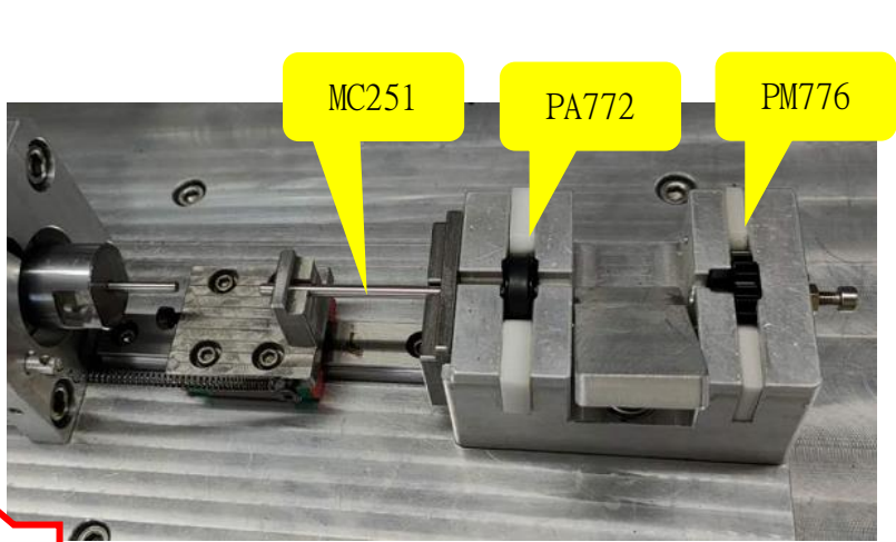
图一，将 PA772,PM776,MC251 装到治具上，确保物料必须放到位，然后关闭防护门，压合完成后将物料处的弹块按压到底取出压好的组件
