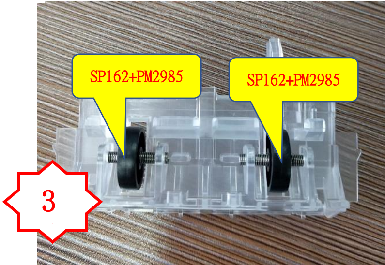
图三，检查组件中 SP162 是否装配到位
