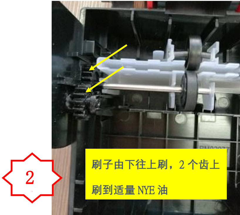
图二，在两个齿轮上刷适量 NYE 油
