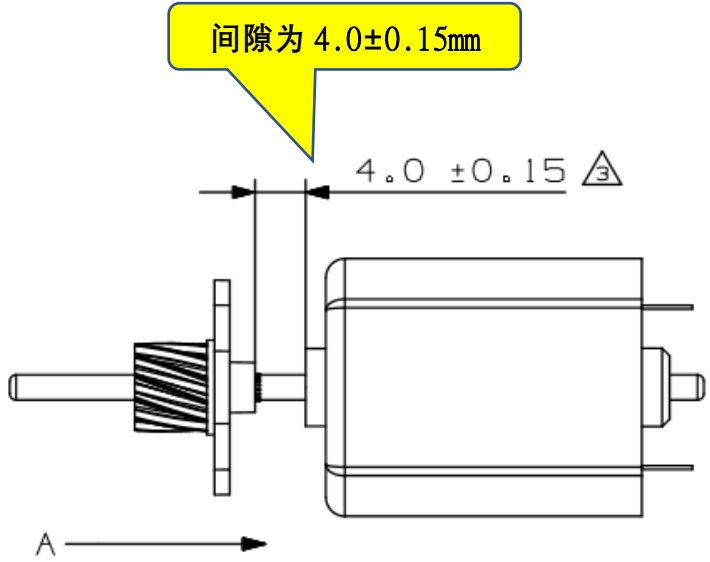
图三， 压合完成后齿轮无损坏， 马达压合后间隙为 4.0±0.15mm
