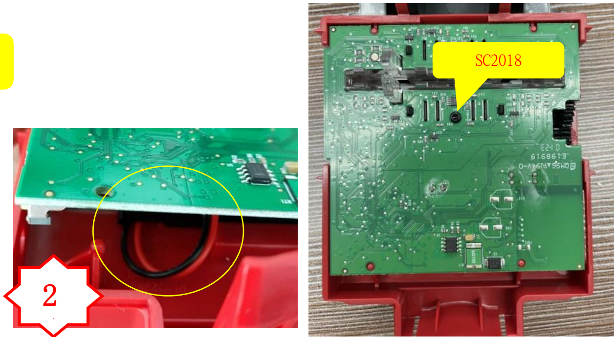
图二，将 PCBA 平放在红色壳子上排好线，打入一颗 SC2018,并打到位
