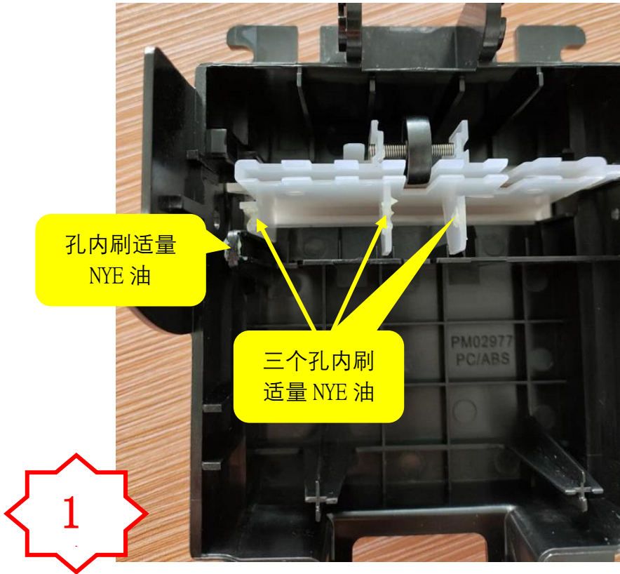
图一，在 PA3363-2 组件的 4 处刷适量的 NYE 油
