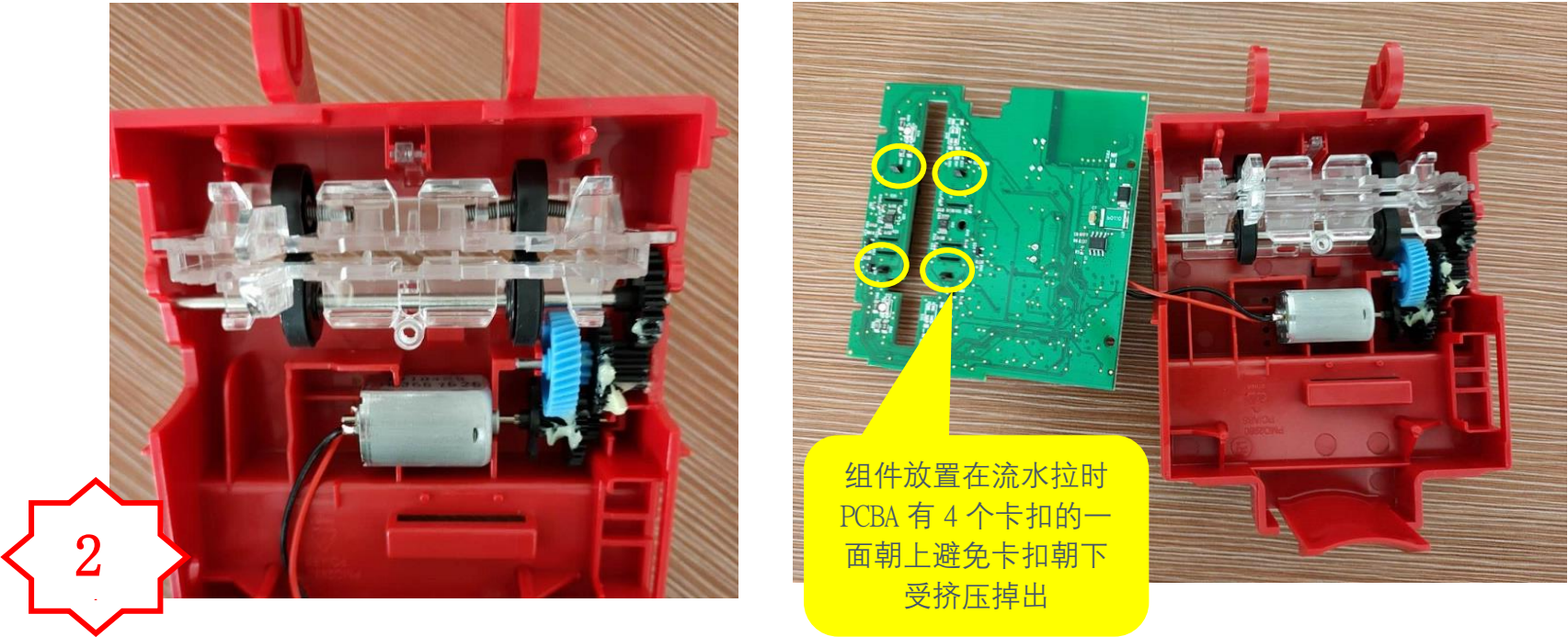
图二，马达有字的一面的一面朝透明组件, 马达需装到底部
