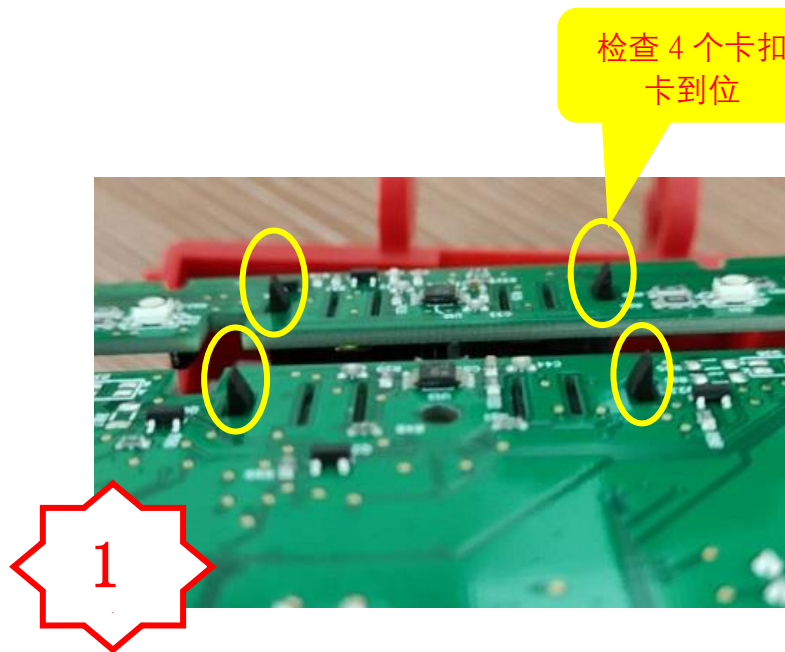
图一，PCBA 上的 4 个卡扣需扣到位
