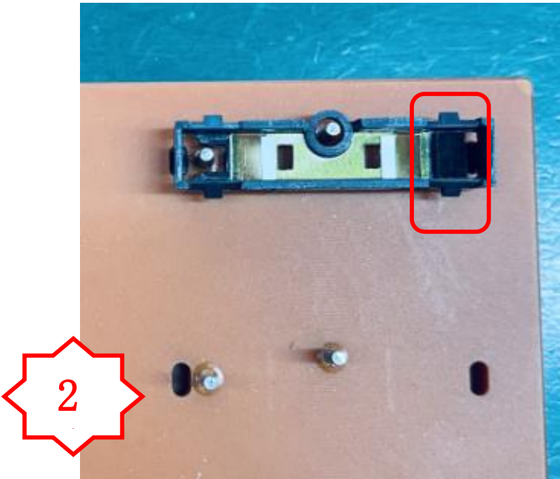
图二，PM2983 螺丝孔朝上放置，将 OP2021 装到组件右边
