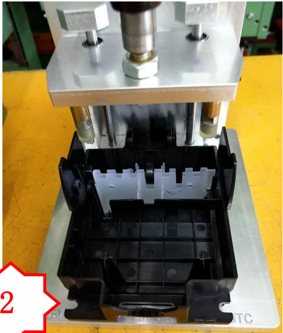
图二，将图二的组件对准 PM2977 两侧的槽位并放到治具上进行压合，注意 PA3365-1 组件的装配方向
