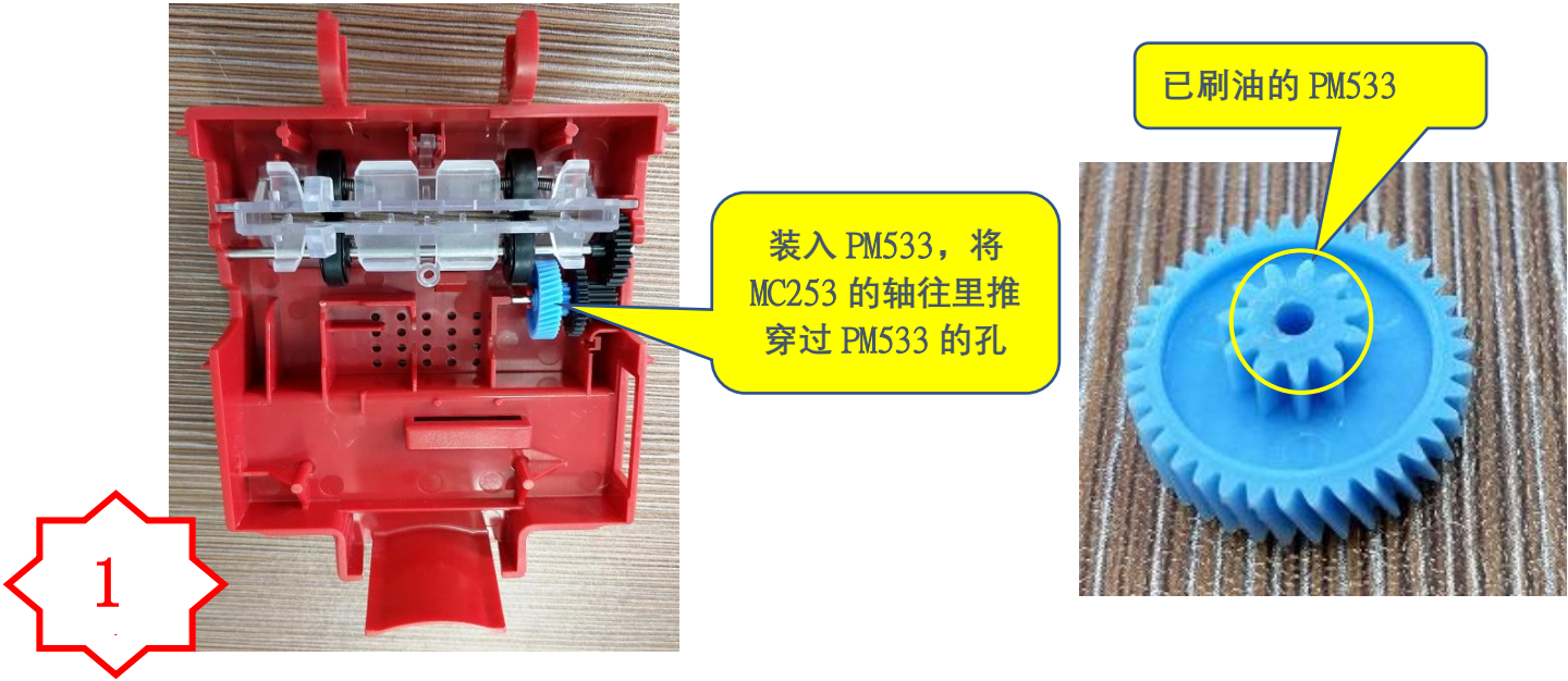
图一，装入 PM533，将轴穿过 PM533 的孔
