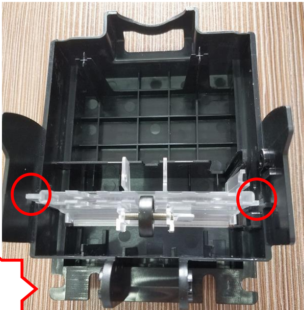
图三，检查两边的卡扣位是否按压到位
