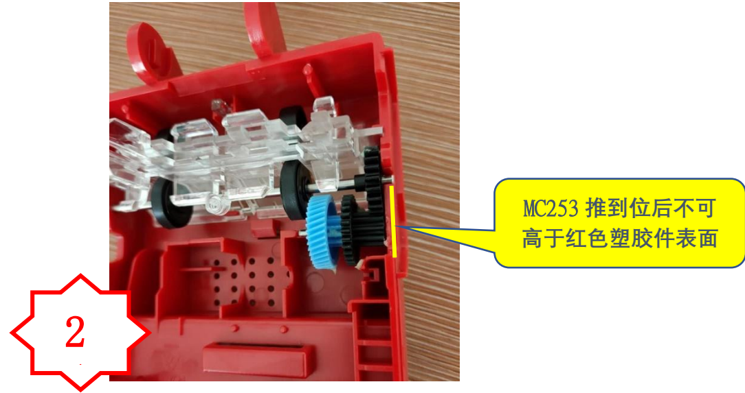
图二，MC253 装到位后不可比红色塑胶件表面高
