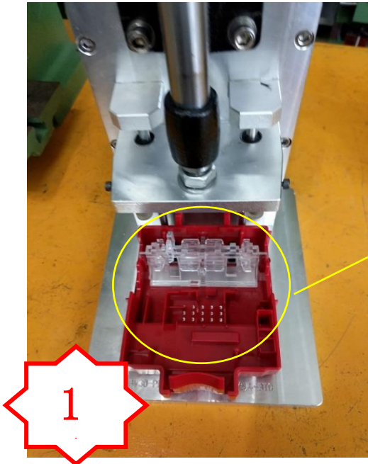
图一，将 PA3365-5 和 PM2984 对准 PM2980 的槽位后用治具压合到位
