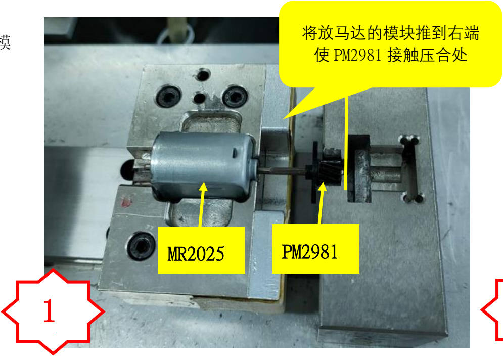
图一， 将 PM2981 扇叶朝马达压合到 MR2025
