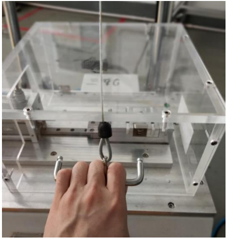
图一，将 PA772,PM776,MC251 装到治具上，确保物料必须放到位，然后关闭防护门，压合完成后将物料处的弹块按压到底取出压好的组件
