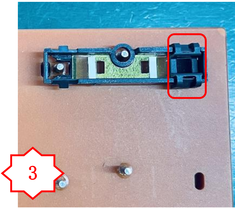
图三，在 OP2021 上装入一个 PM3011，卡扣朝下装入,注意两侧卡扣需扣到位
