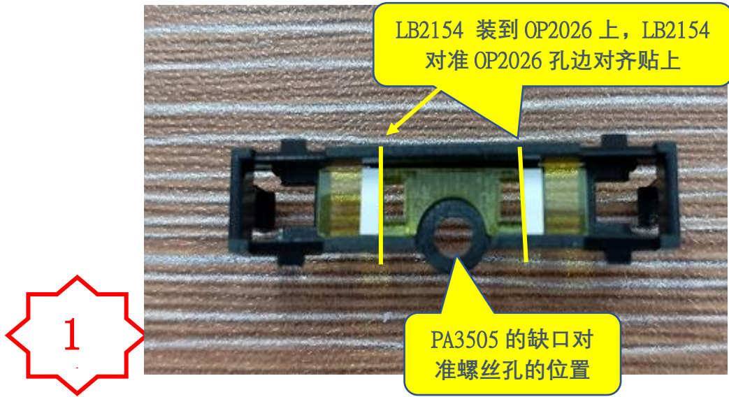
图一，将 2 个 LB2154 贴到 OP2026 上，贴平 OP2026 窗口的边
