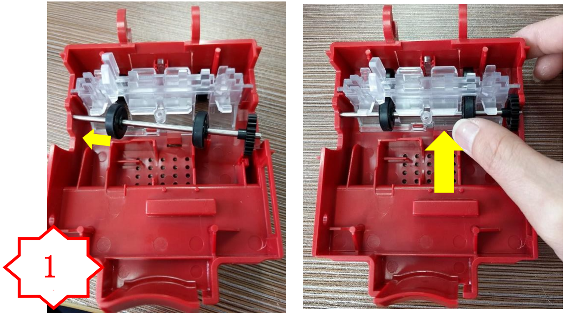
图一，将 PA773 的一侧装到孔内，然后按压中间的轮子装配到位
