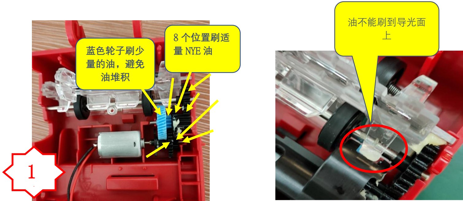
图一， 在图上 8 个位置刷 NYE 油，注意油不能刷到导光柱上
