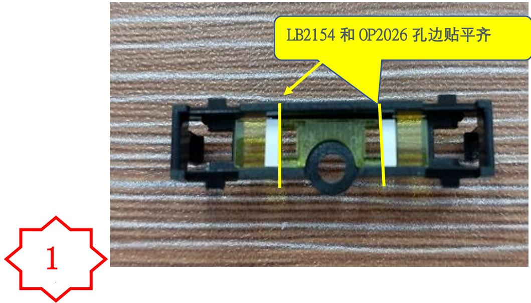
图一，贴好 LB2154 的组件
