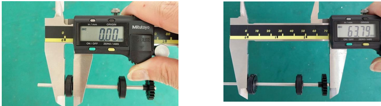
用卡尺卡住 PA772 后将卡尺归零，然后按照上图位置测量
