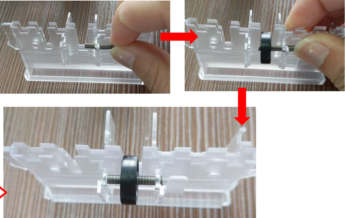
图二，将 SP162 先装到 PM2978 的一侧孔内，再将 PM2985 装在 SP162 上，然后将 SP162 推到另一孔内
