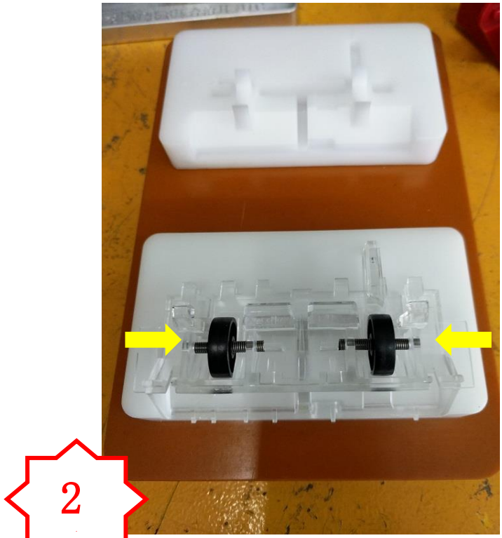
图二，穿入 2 个 SP162 到 PM2979 底端
