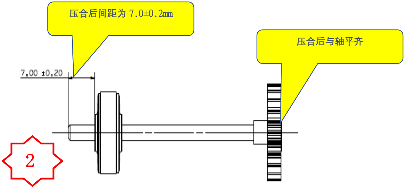
图二，将 PM776 和 PA772 压合到 MC251 上
