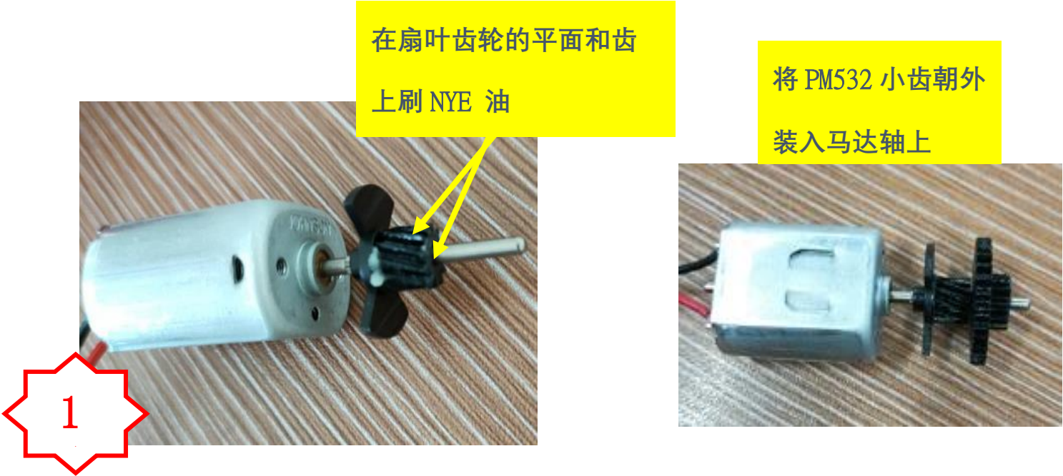
图一，在马达扇叶齿轮的平面和齿的表面刷 NYE 油, 并将 PM532 小齿朝外装入马达轴上
