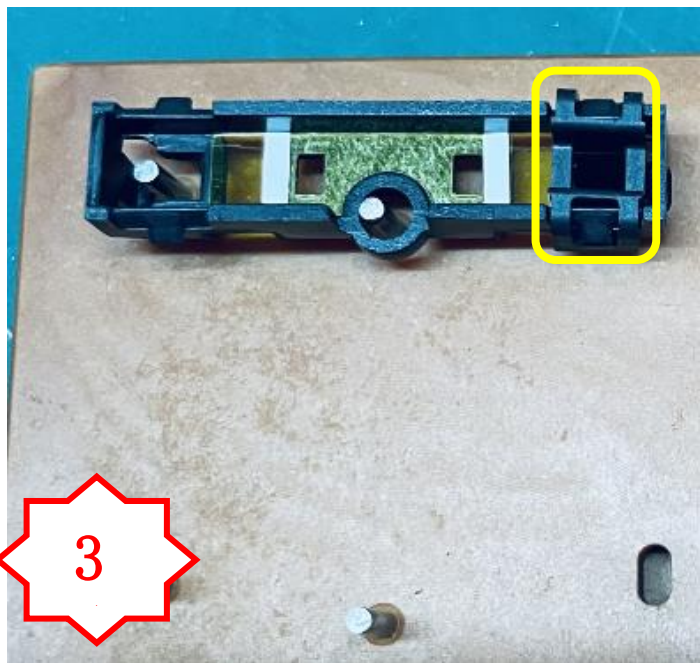
图三，在 OP2021 上装入一个 PM3011，卡扣朝下装入,注意两侧卡扣需扣到位
