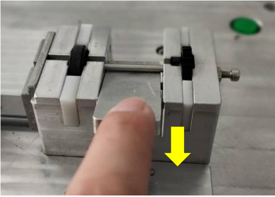
图一，将 PA772,PM776,MC251 装到治具上，确保物料必须放到位，然后关闭防护门，压合完成后将物料处的弹块按压到底取出压好的组件
