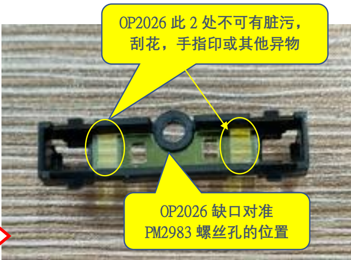
图二，将 OP2026 装到 PM2983 上，OP2026 装到位后贴平 PM2983
