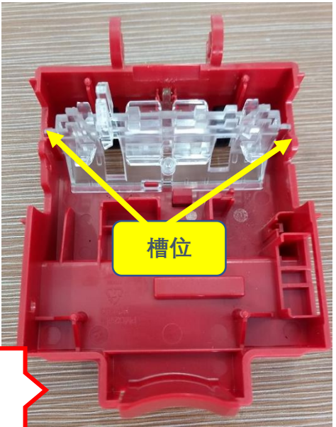
图二，透明组件需对准 PM2980 的槽位
