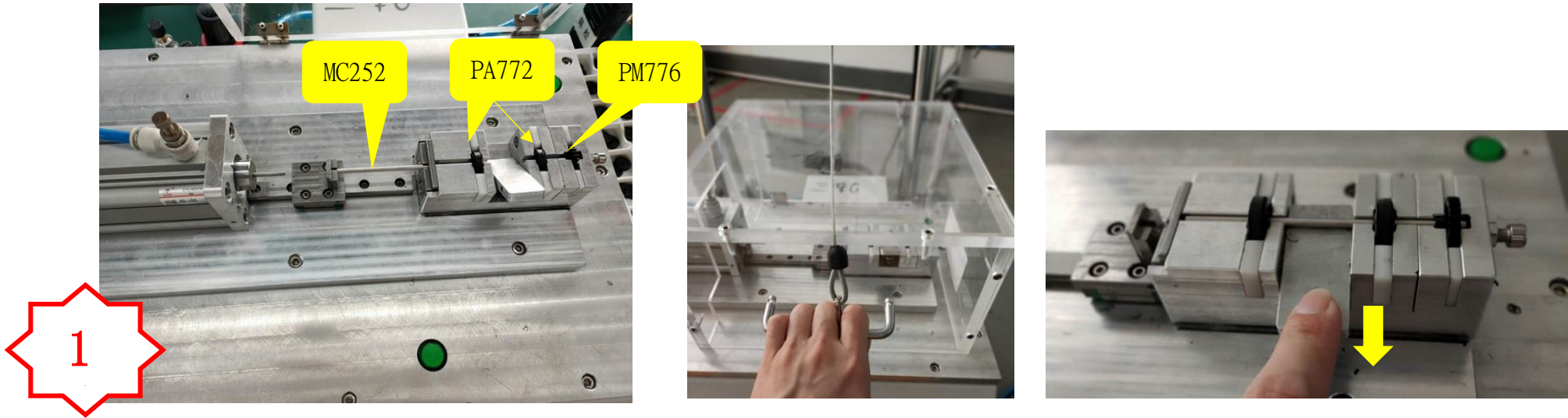
图一，将 2 个 PA772,PM776,MC252 装到治具上，确保物料必须放到位，然后关闭防护门，压合完成后将物料处的弹块按压到底取出压好的组件
