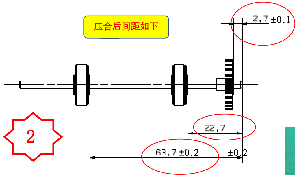
图二，将 1 个 PM776 和 2 个 PA772 压合到 MC252 上，确保尺寸符合上图要求
