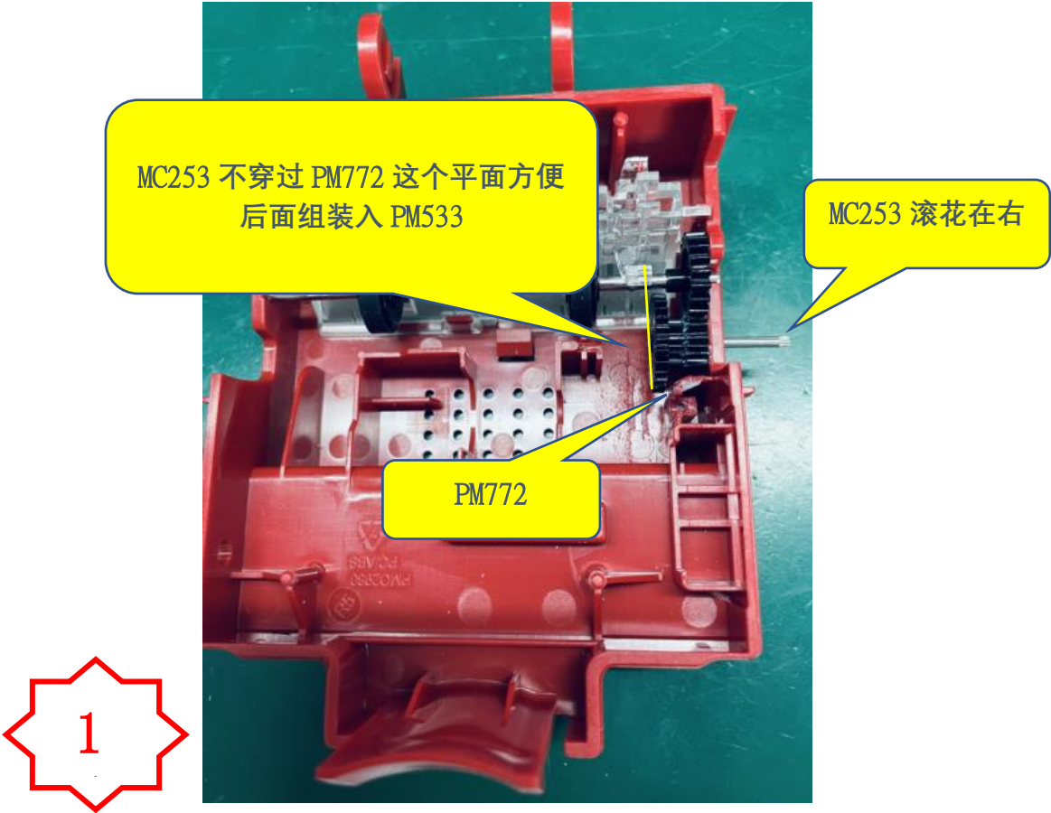
图一， 将 MC253 穿入一个 PM772， 注意 MC253 滚花在右
